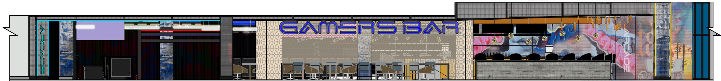
1 WEST ELEVATION Scale: 1/8" = 1'-0"
